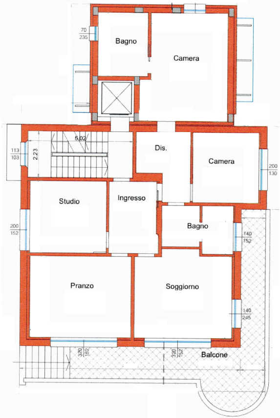
PIANO Primo H. mt.3.43
