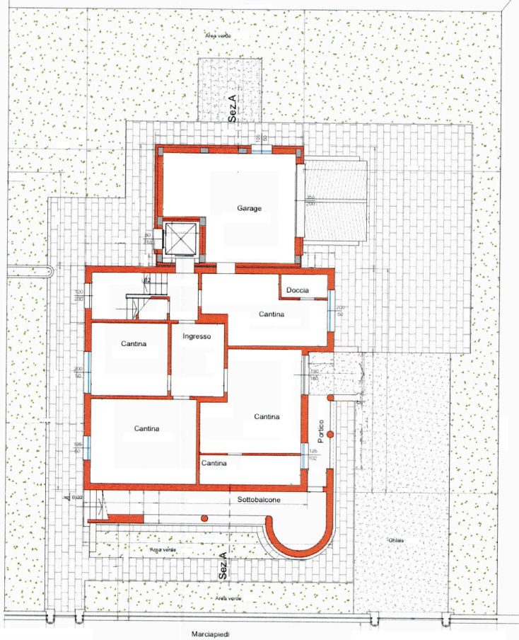
PIANO Terra H. mt.2.18
